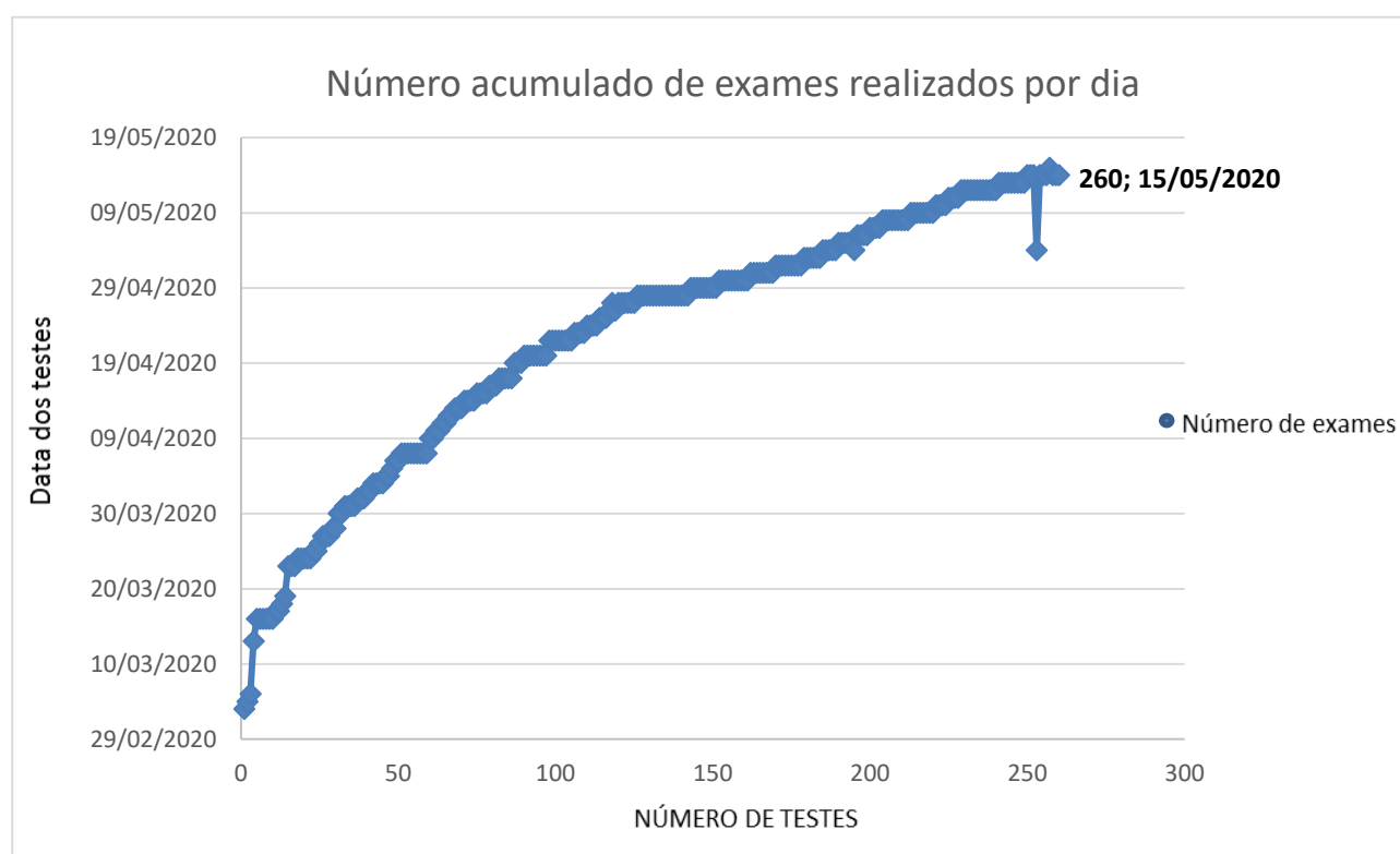
Gráfico1. Número acumulado de exames coletados para SARS-COV2 entre 04/03/2020 a 15/05/2020. Um total de 260 coletas foram realizadas em 226 pacientes.
