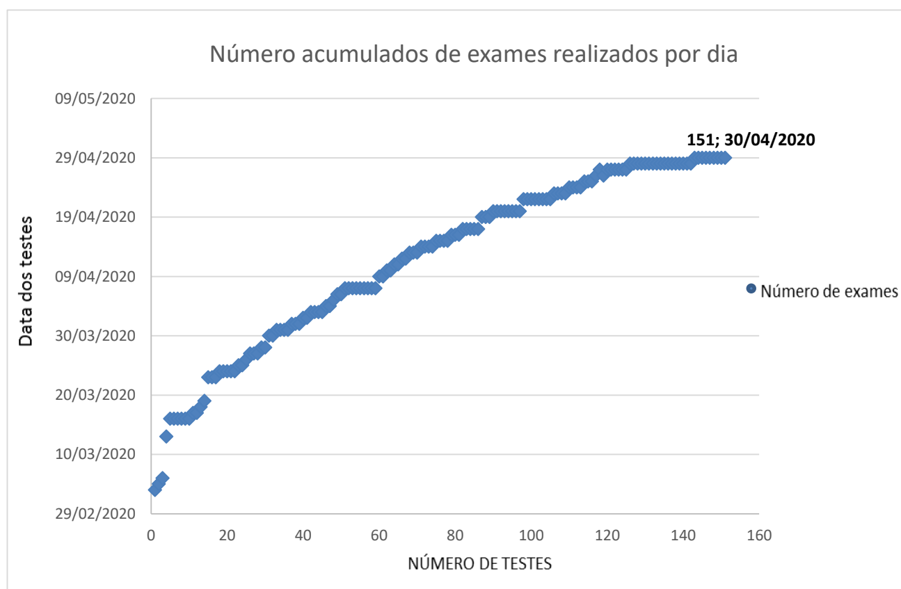
Gráfico 1. Número acumulado de exames coletados para SARS-COV2 entre 04/03/2020 a 30/04/2020. Um total de 151 coletas foram realizadas em 132 pacientes.
