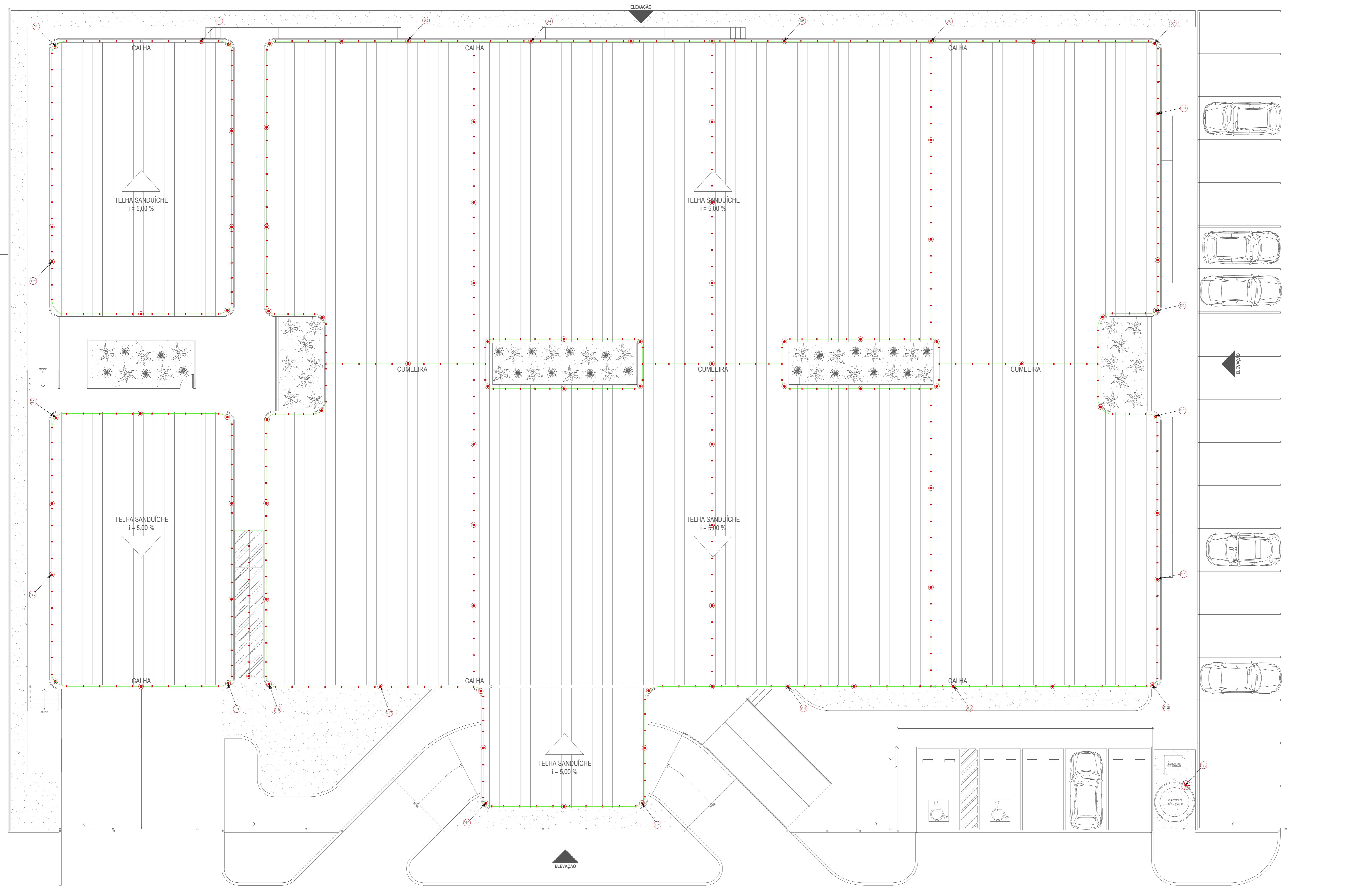
PLANTA DE COBERTURA - SPDA UNIDADE DE PRONTO ATENDIMENTO - PORTE 3 EDIFICAÇÃO TIENHA E=1:100
