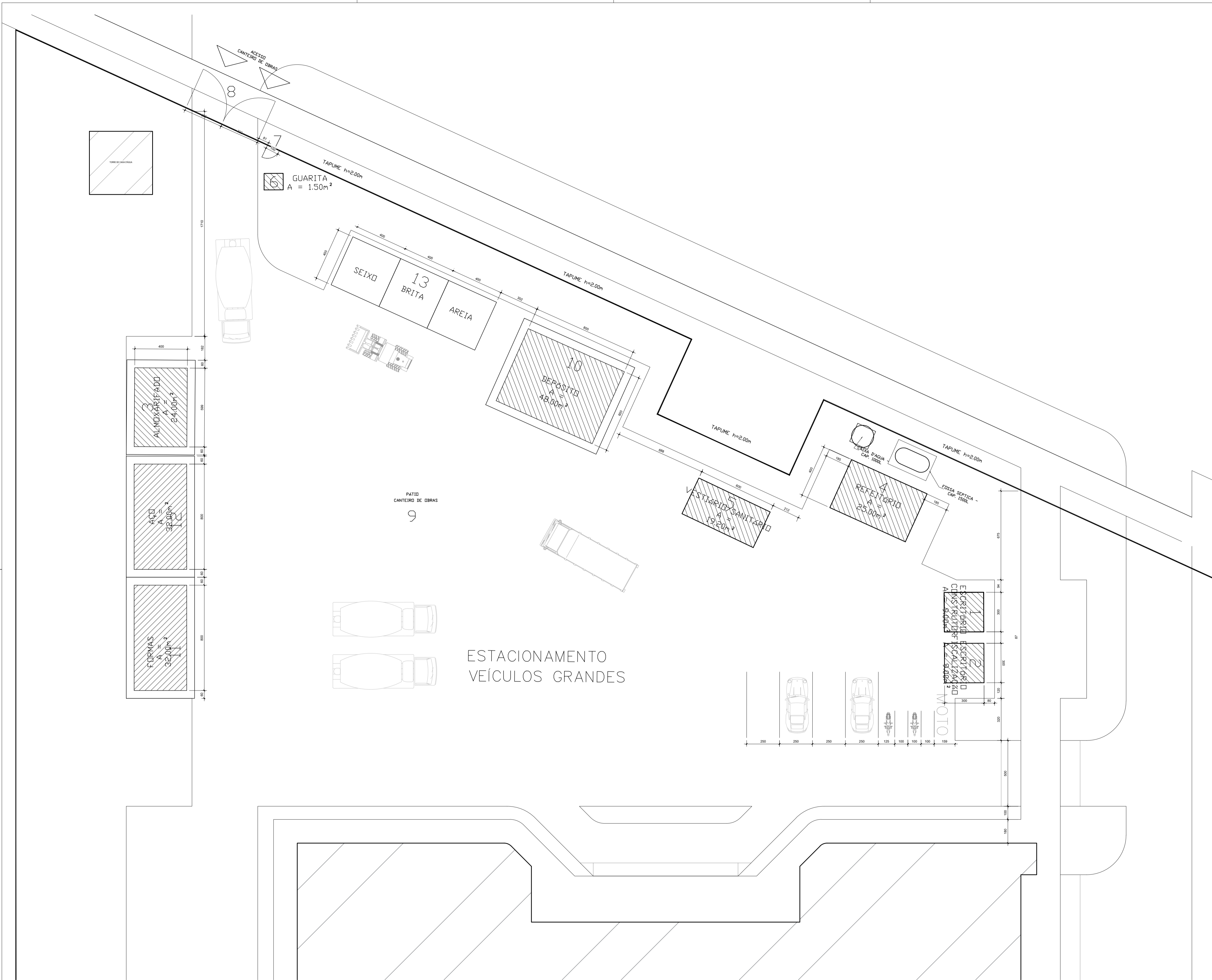
PLANTA DE LOCAÇÃO CANTEIRO DE OBRAS Escala: 1 : 150
